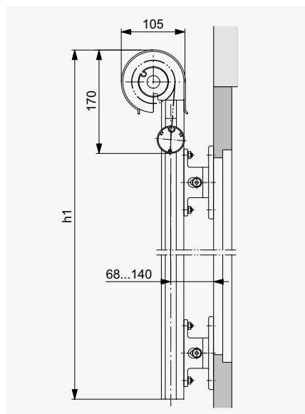
Rieles guía
