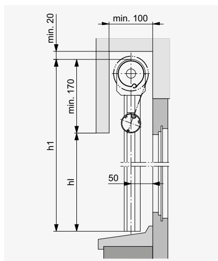
Rieles guía
