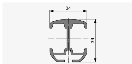
Guía doble
